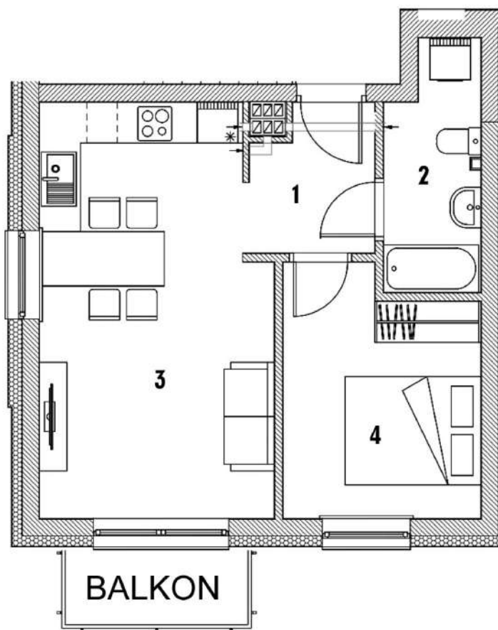
RZUT KONDYGNACJI 3 POZIOM 1 PIĘTRO
