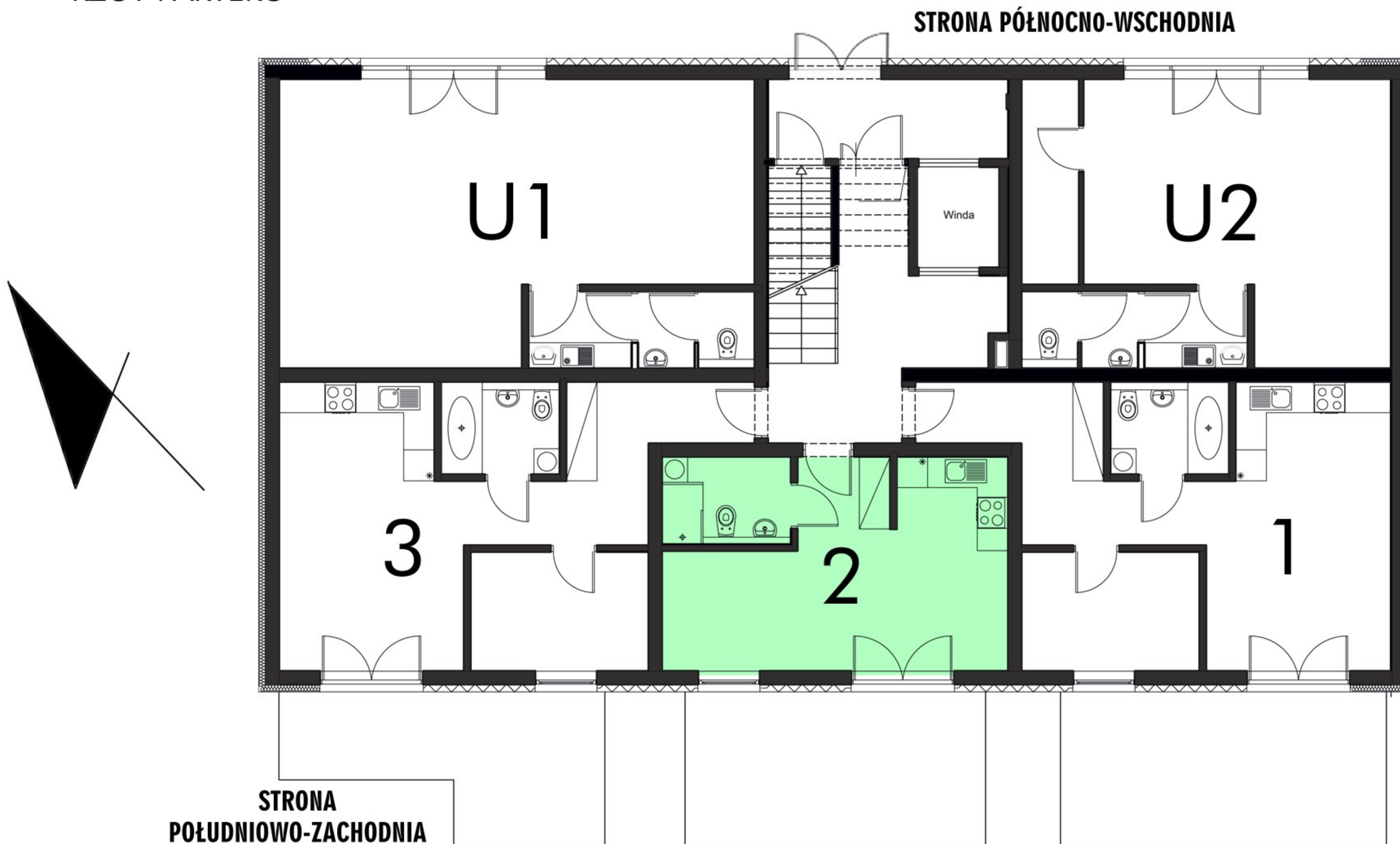
RZUT PARTERU
